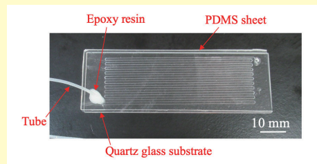
マイクロ流路デバイスの試作
