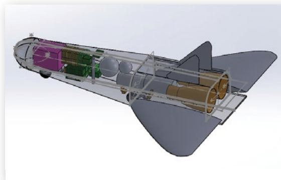
●有翼宇宙往還機の概念検討
