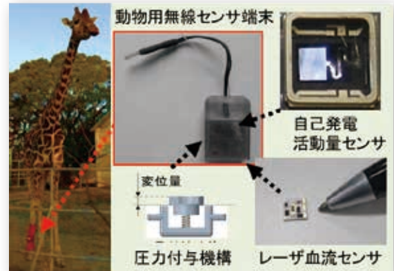
●MEMSと機構を活用した装着型センサ
