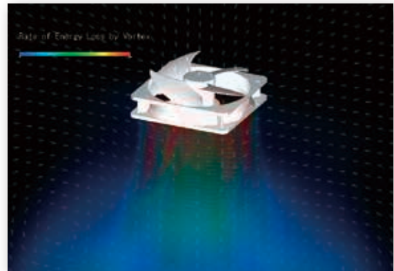
●数値解析による空冷用ファンの渦損失構造の可視化
