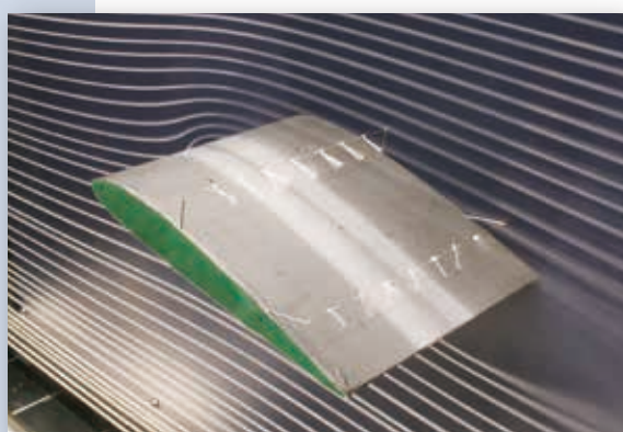
●翼まわりの気流可視化風洞実験
