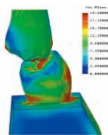
●歯の咬合による応力分布解析 (FEM)
