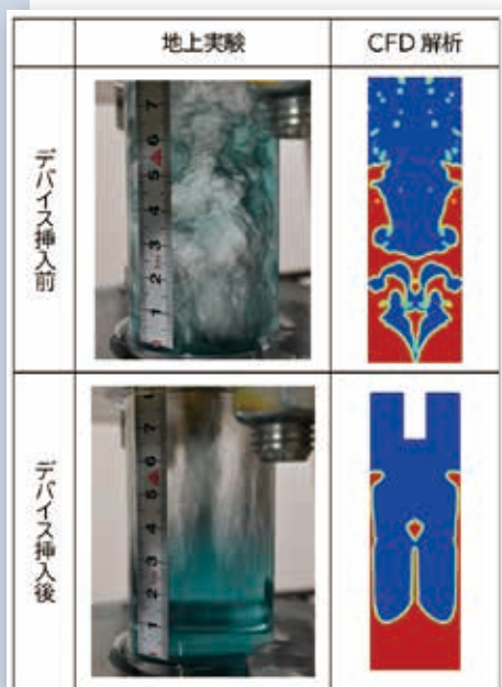
●宇宙機推進薬タンク内液面挙動
