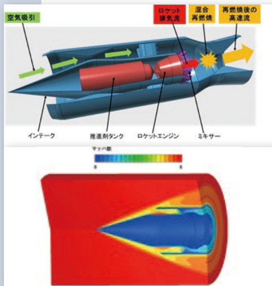
●ラムロケットエンジン内部のCFD解析
