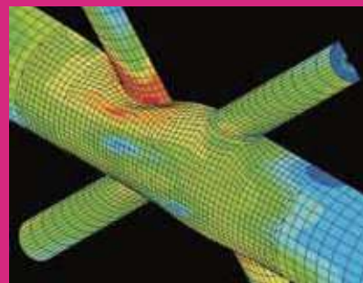
接合部の解析例(鋼管接合部) 数多くの実験と解析(3Dシミュレーション)を行うことで、的確に破壊の予測が可能であることが示された。
